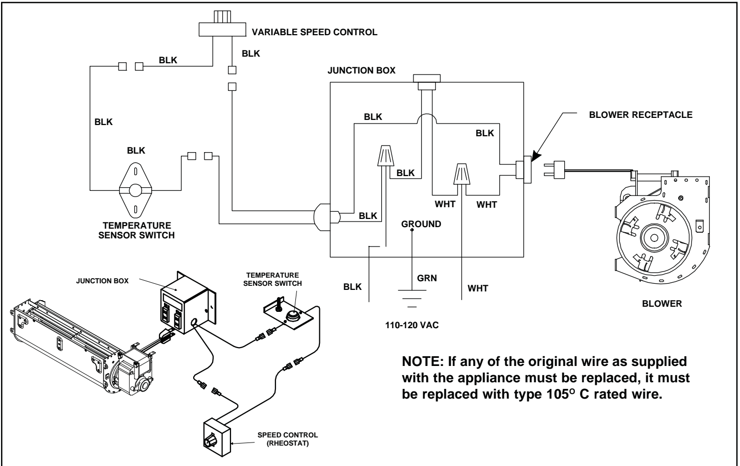
Figure 27. Fan Wiring Diagram
