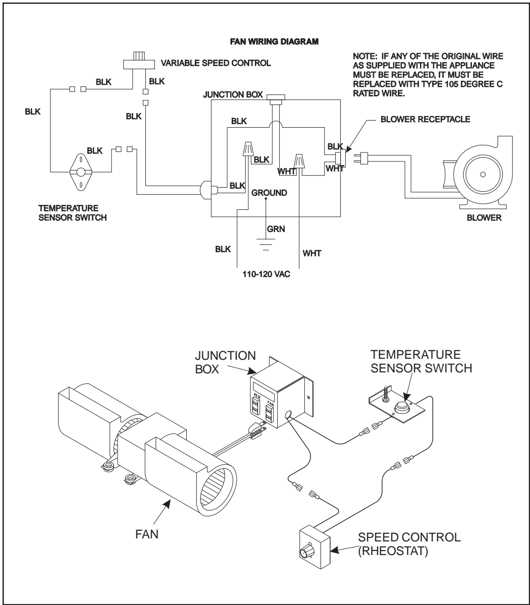
Figure 26. Fan Wiring Diagram
