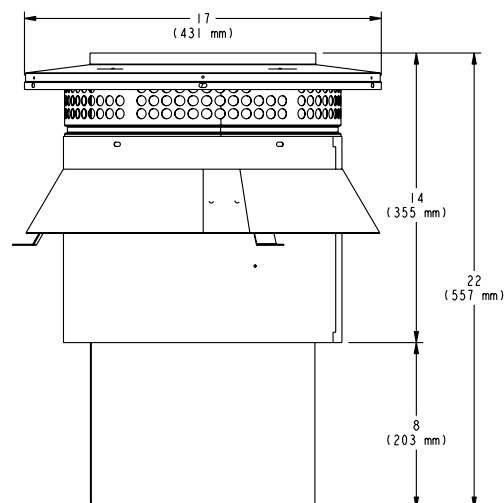
CT11-A Adapter
