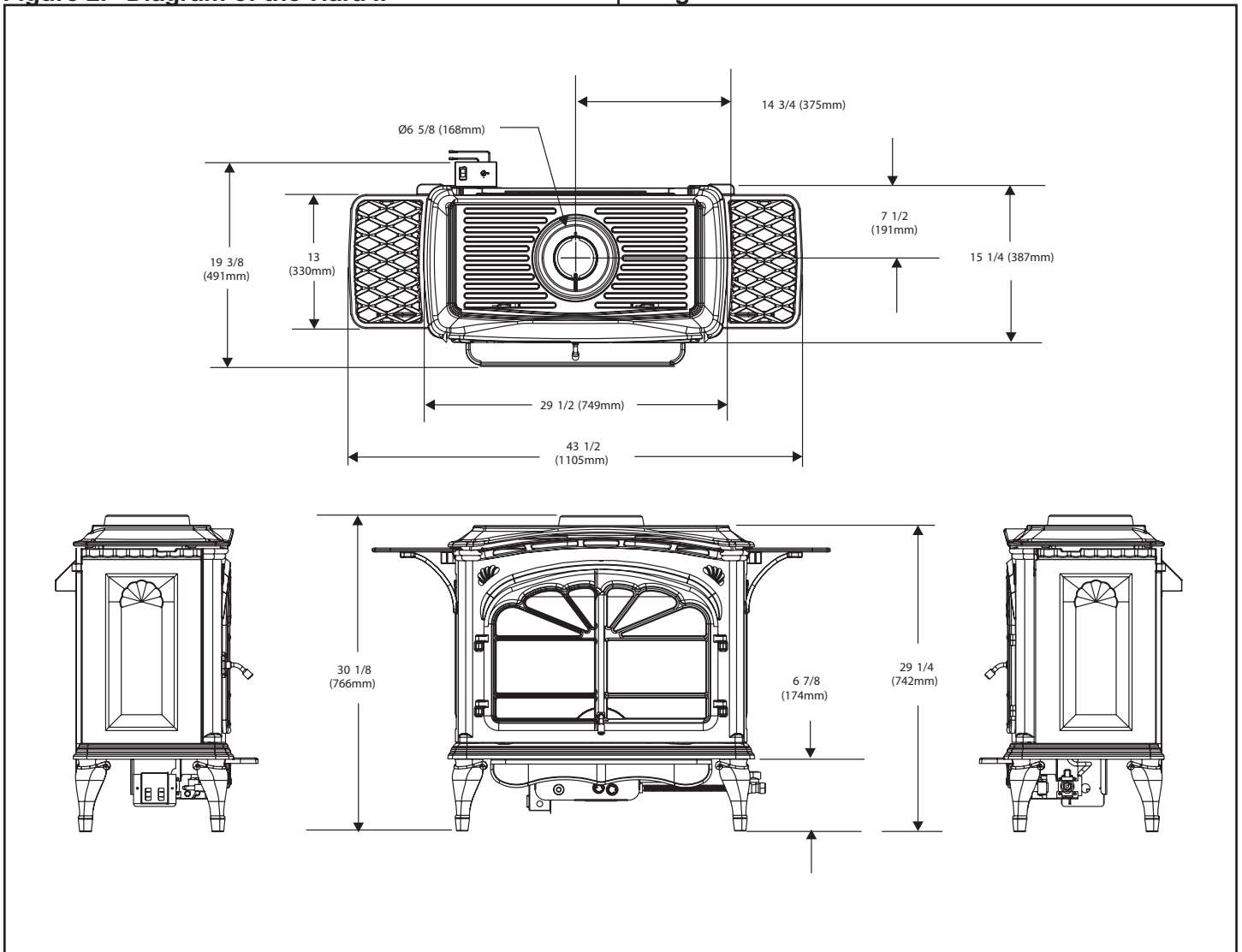
Figure 2. Schéma du modèle Tiara II
