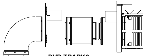
DVP-TRAPK2
