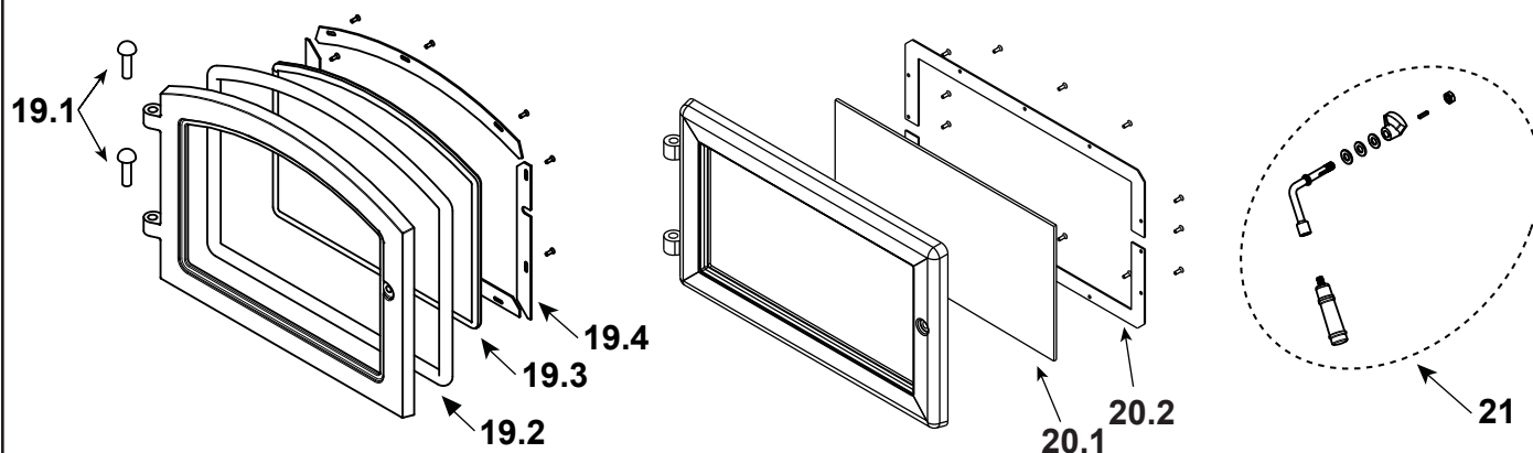
#19 Arch Door Assembly
