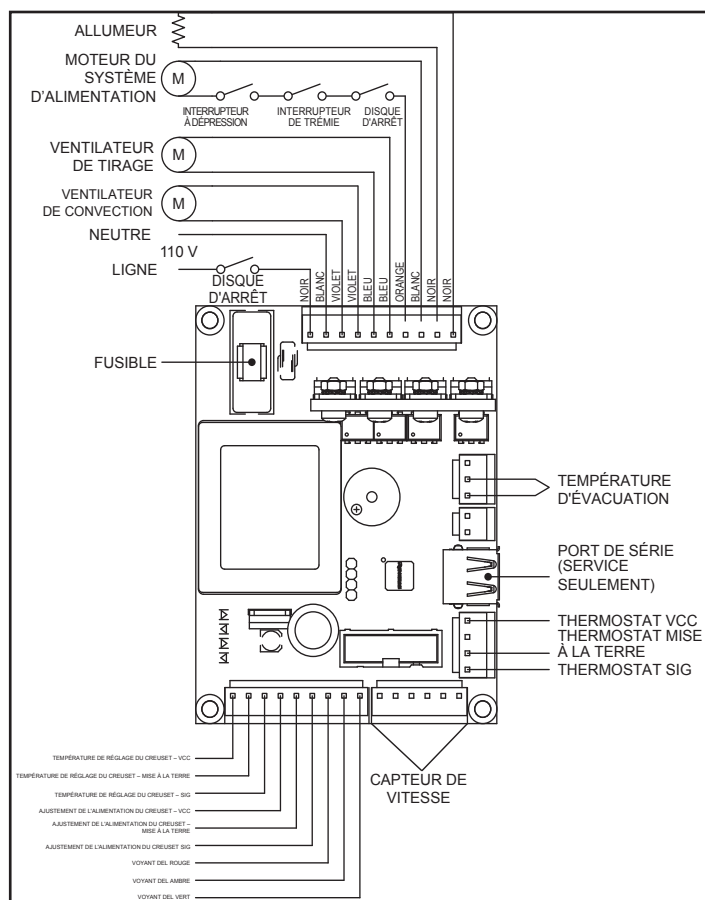
Figure 28.1 – Schéma de la carte de commande
