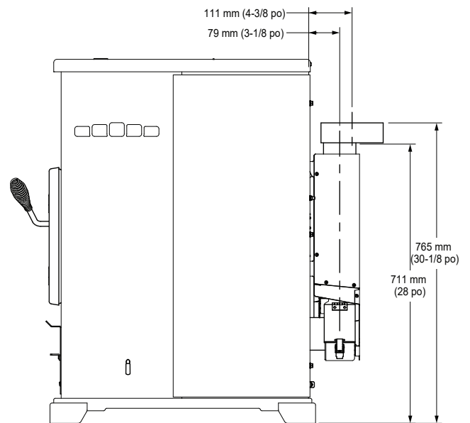
Figure 8.4 – Vue latérale avec adaptateur supérieur de ventilation
