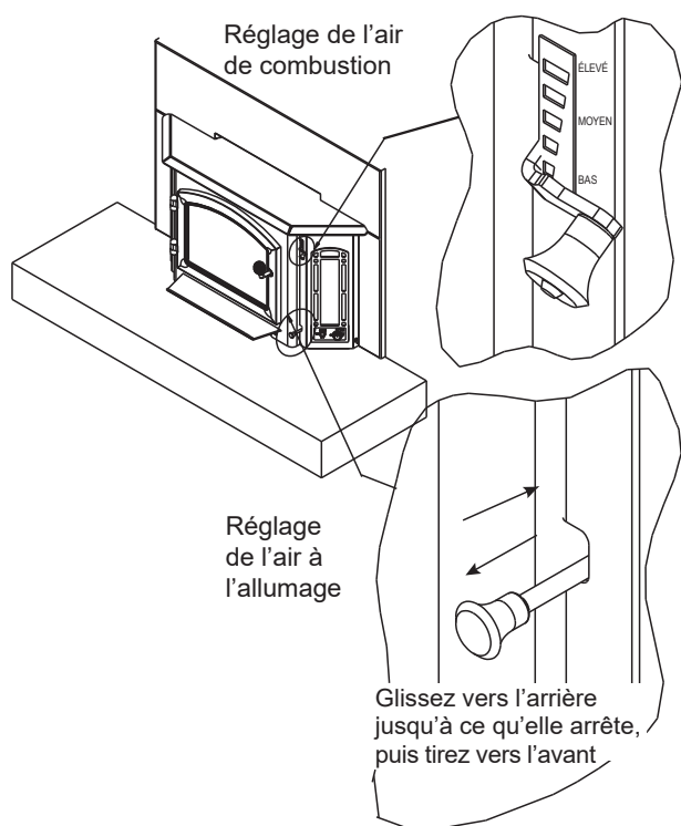
Figure 13.1 - Réglages de l'air à l'allumage et de combustion
