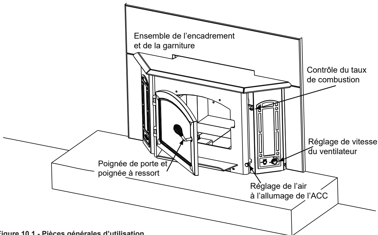
Figure 10.1 - Pièces générales d'utilisation
