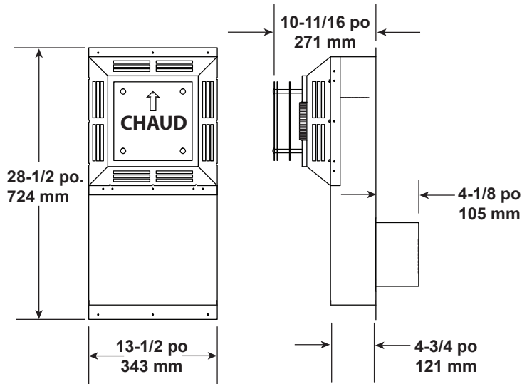
SLP-CCS-BK Boîte support pour plafond cathédrale – noire
