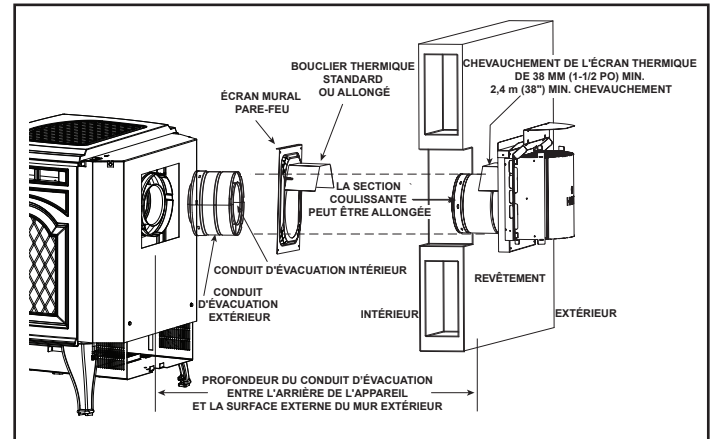
Figure 7.17 Évacuation à travers le mur
