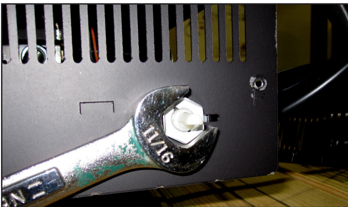
Figure 8.8 Installer le réglage de vitesse à l'aide de l'écrou Pal
