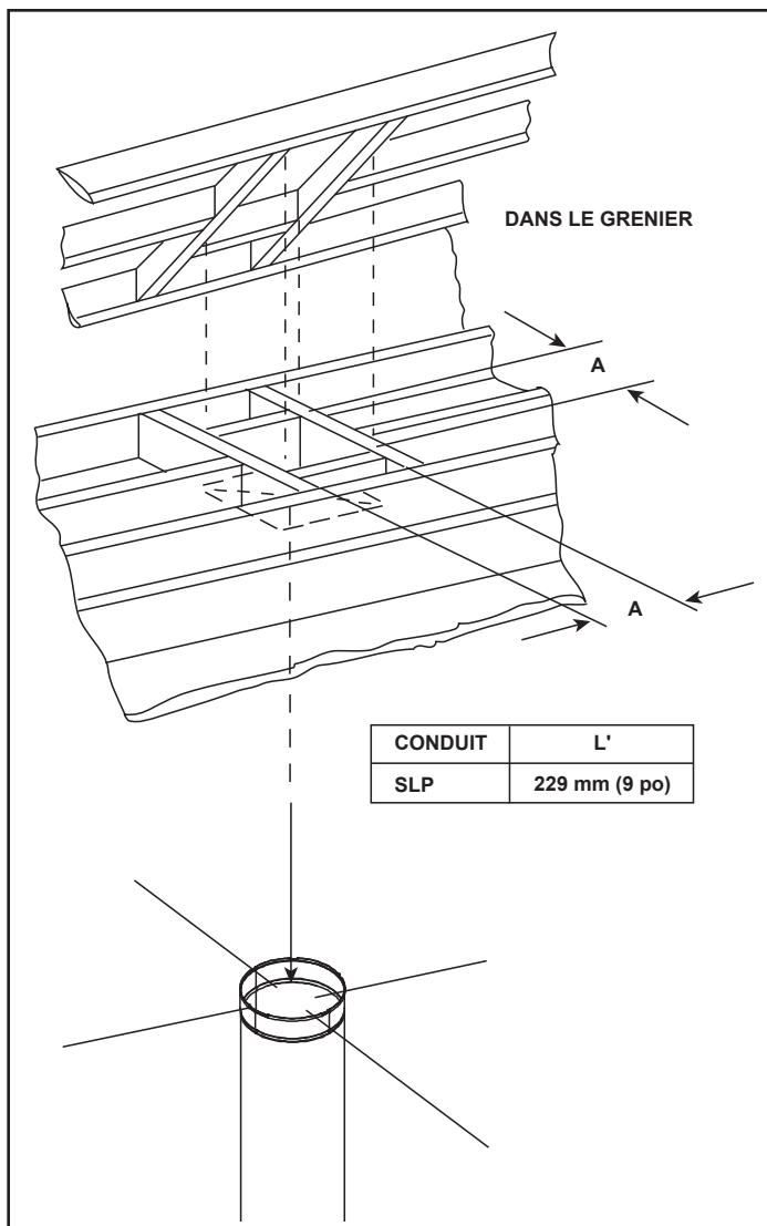
Figure 5.3 Installation du coupe-feu de grenier
