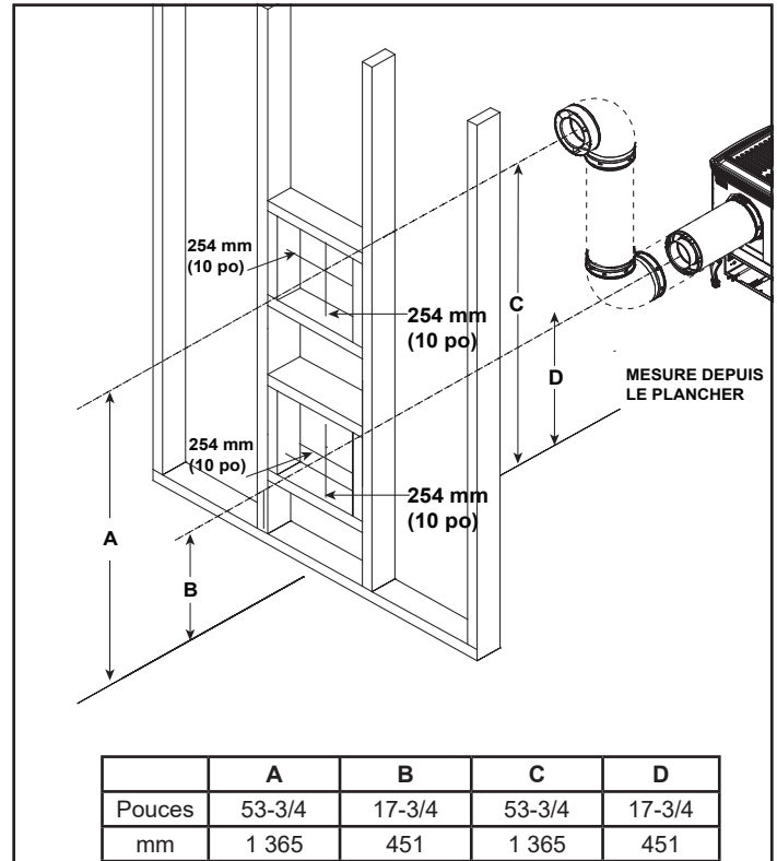
Figure 5.2 Pénétration du mur
