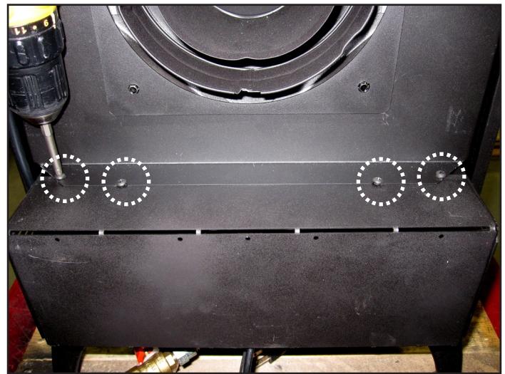
Figure 8.5 Fixer le ventilateur avec quatre vis
