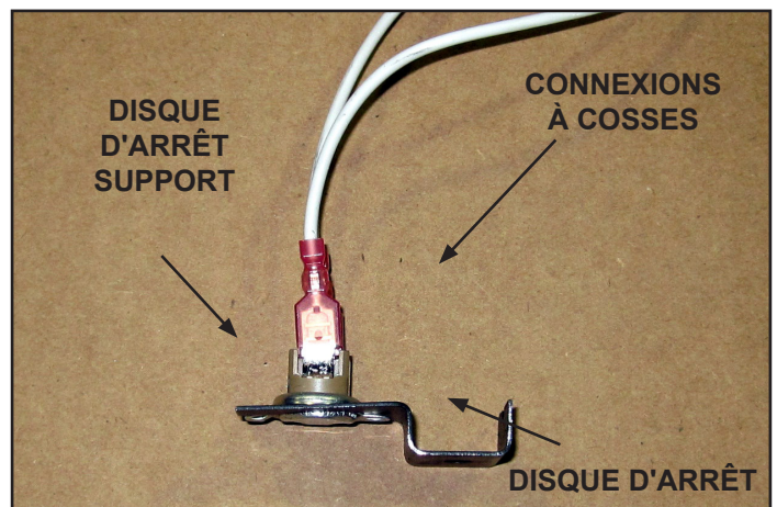
Figure 8.6 Installer le disque d'arrêt
