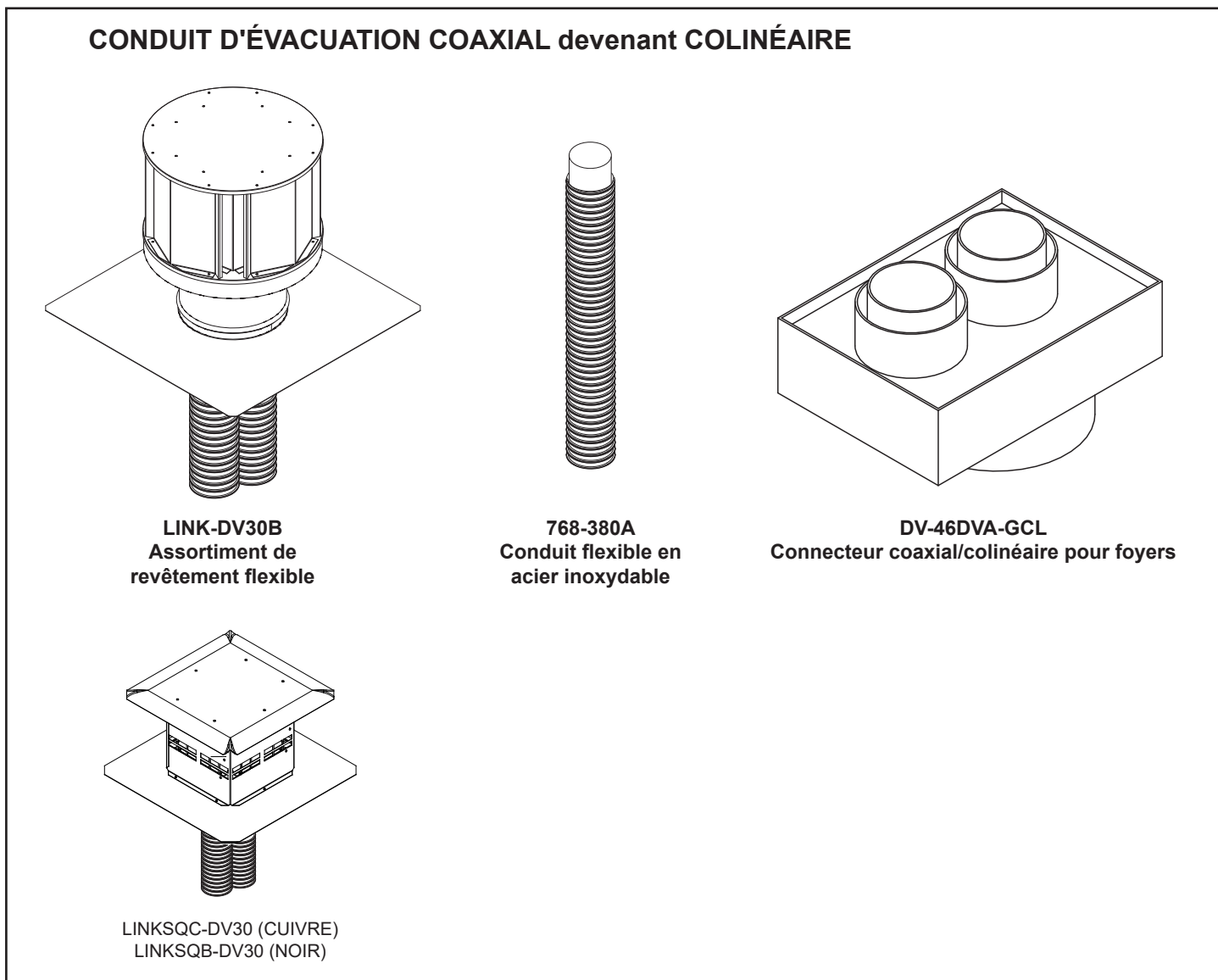
Figure 11.4 Composants du conduit de série SLP
