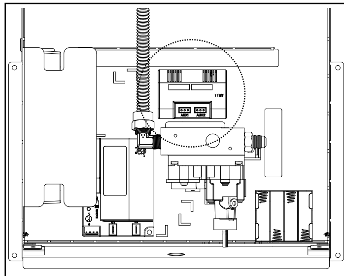
Figure 8.3 Boîte auxiliaire
