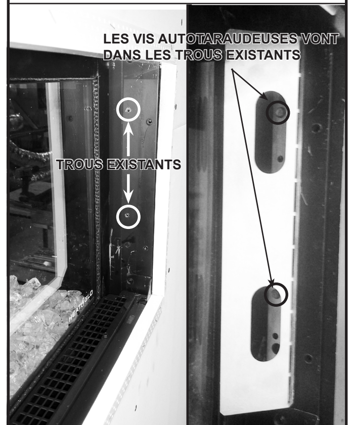
Figure 10.15 Installer le support du panneau de verre de transition
