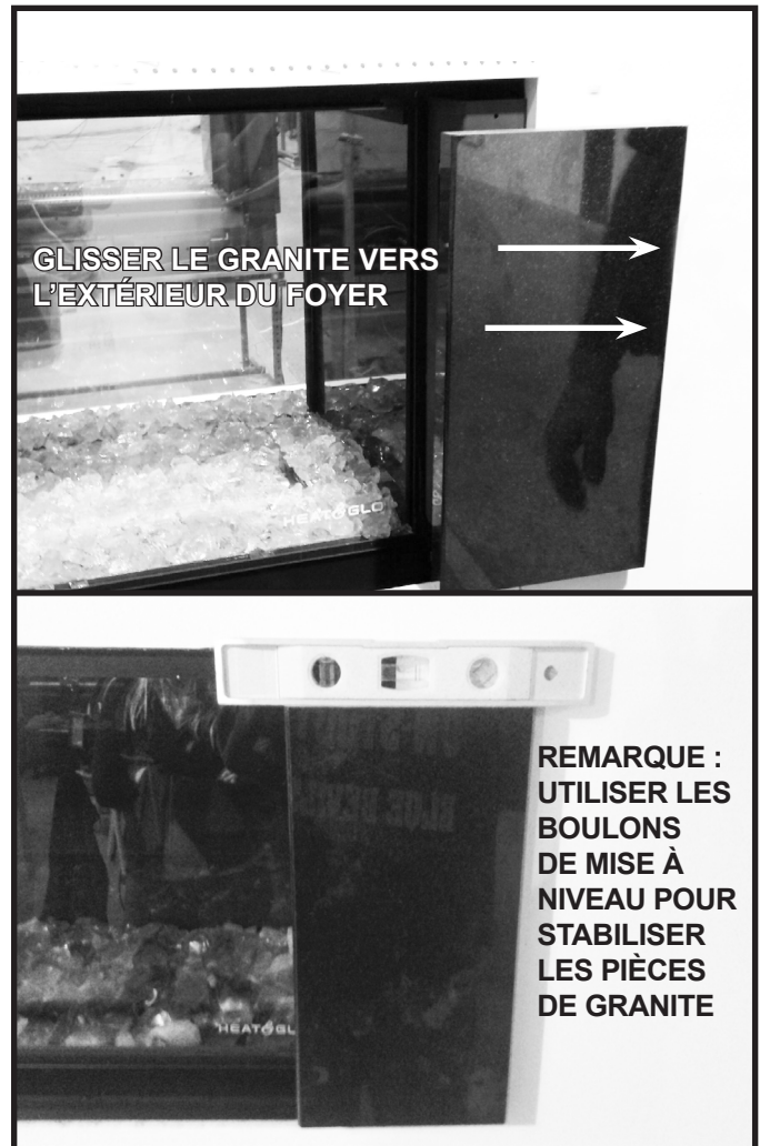
Figure 10.26. La pièce de granite de droite est installée et mise à niveau
