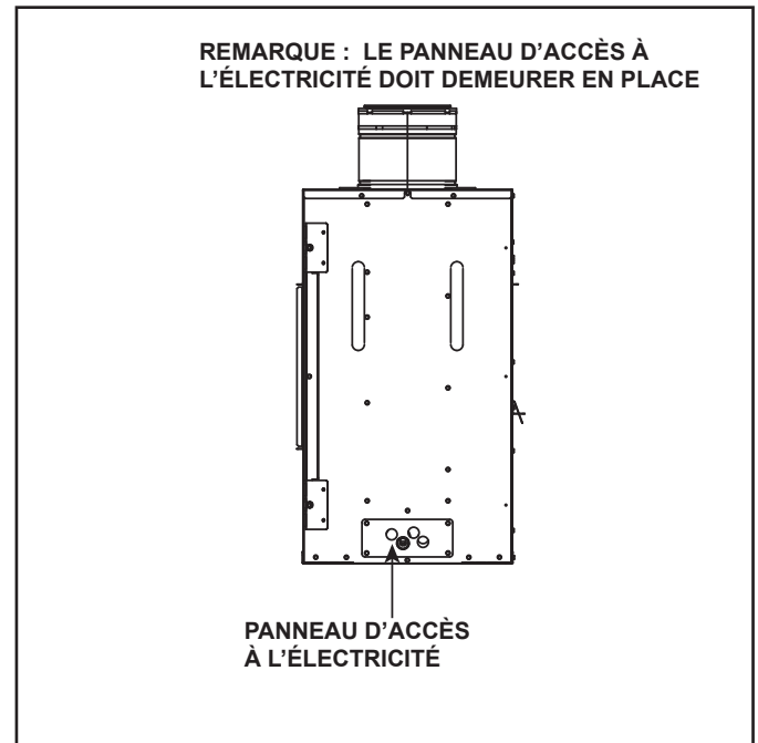
Figure 9.8 Emplacement de l'accès électrique – côté droit
