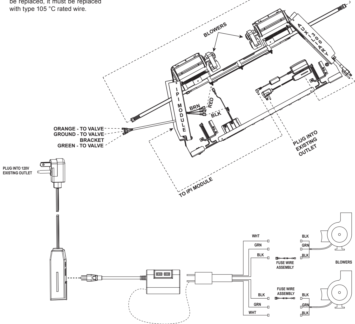
Figure 8.2 Fan Wiring Diagram
