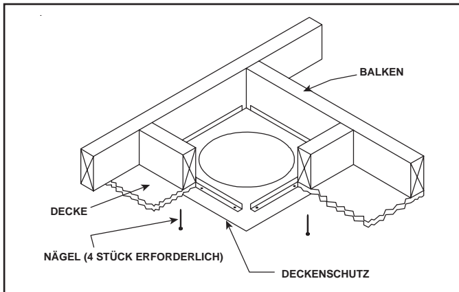
Abbildung 10.12 Deckenschutz (deckenseitig)
