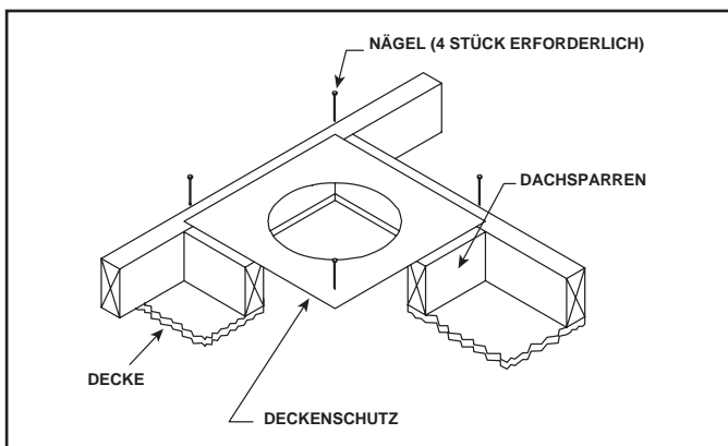
Abbildung 10.13 Dachbodenschutz
