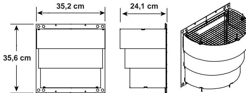
DRC-RADIUS Schutzvorrichtung für Mündungselement
