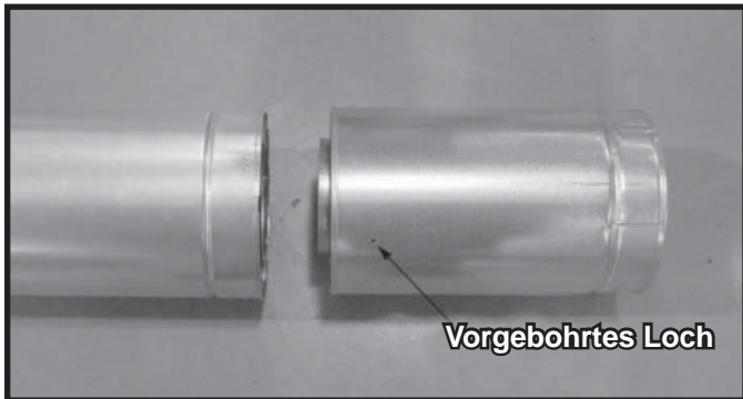
Abbildung 10.3 Vorgebohrte Löcher im Gleitelement
