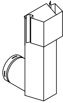
SLK-SNKD Schacht-Mündungselement
