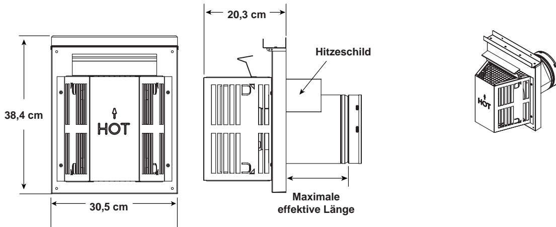
SLP-TRAP Horizontales Mündungselement
