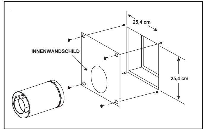
Abbildung 10.10 Abzugsrohr und Wandschutz
