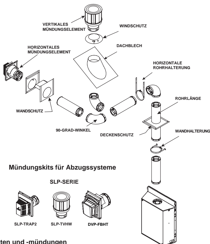
Abbildung 7.8 Abzugskomponenten und -mündungen
