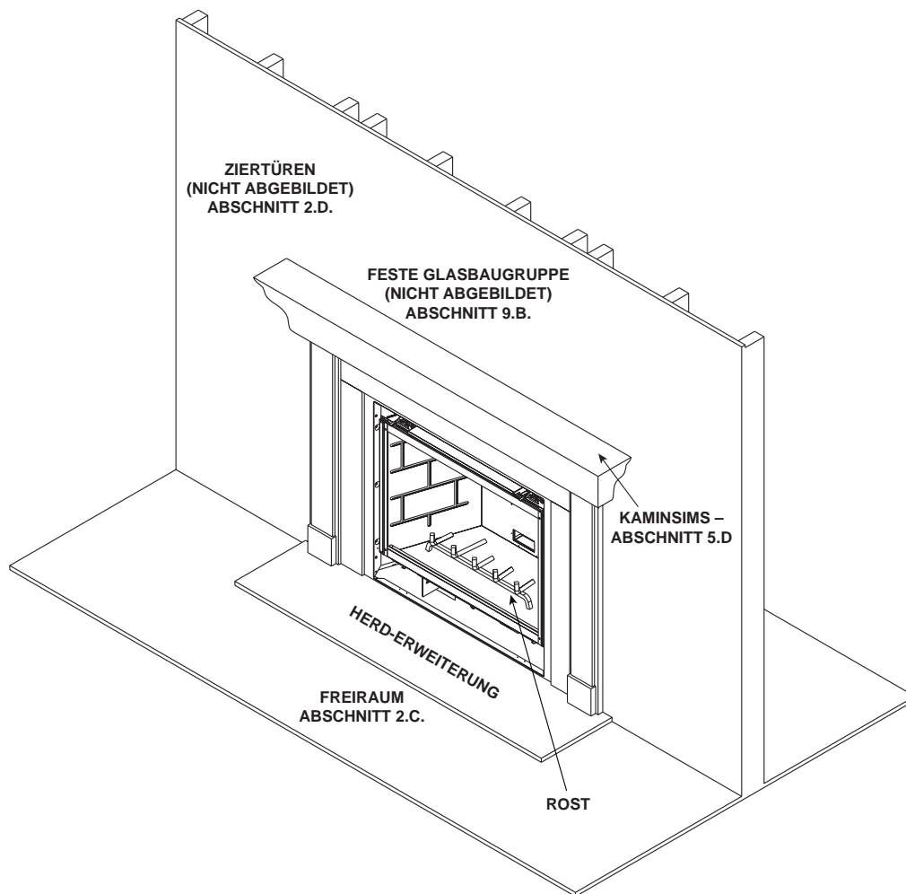
Abbildung 2.1 Allgemeine Funktionsteile
