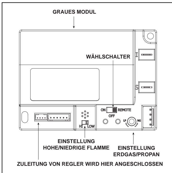
Abbildung 2.3 Steuermodul
