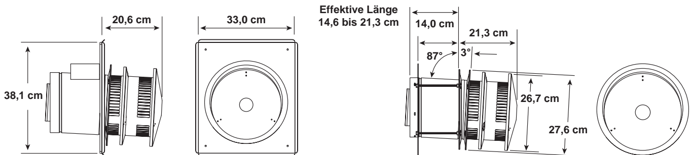
SLP-HRC-SS SLP-HRC-ZC-SS Horizontales mündungselement
