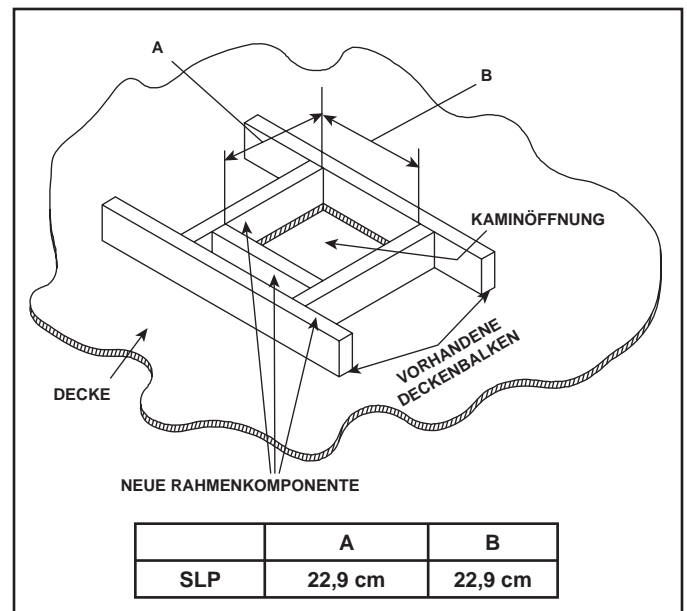
Abbildung 10.11 Öffnung und neue Rahmenkomponenten
