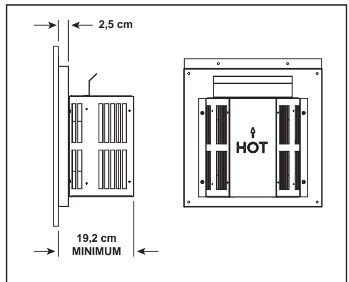
Abbildung 10.15 Mündungselement
