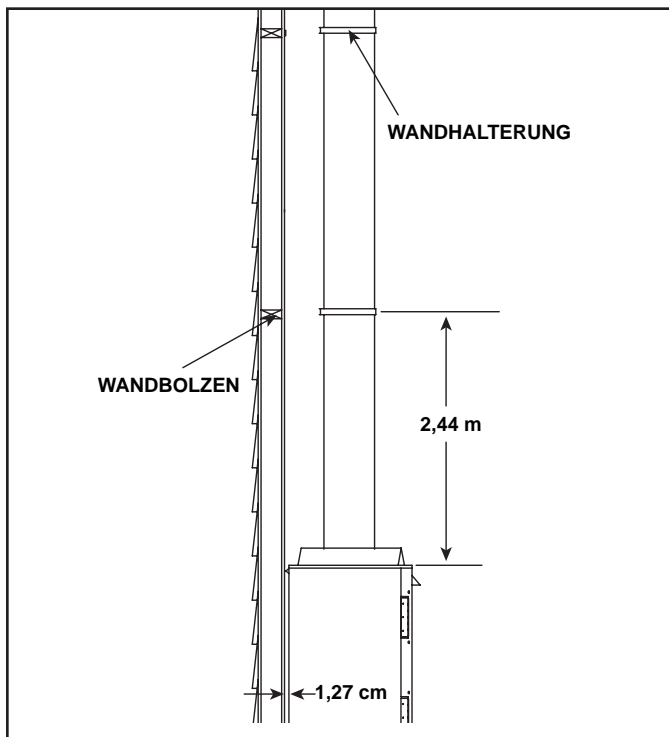
Abbildung 10.9 Installieren der Halterungen
