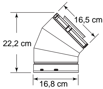
SLP-45 - 45°-Rohrkrümmer
