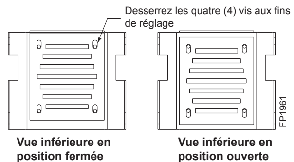
Figure 17 - Ensemble de chicane et réglage
