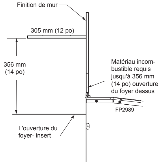
Figure 4 - Dégagements du manteau
