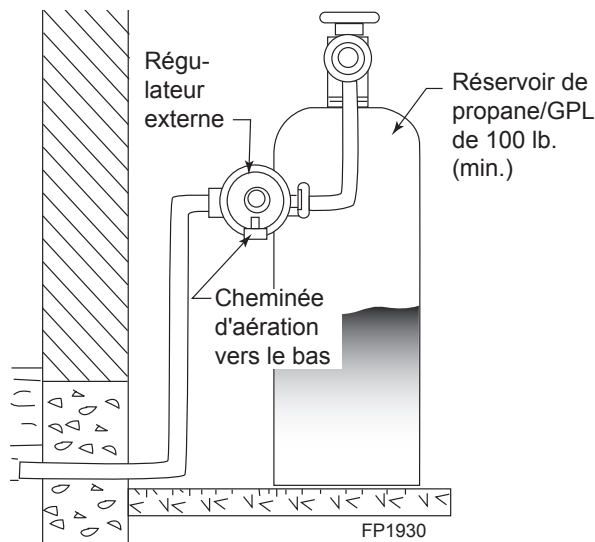
Figure 18 - Régulateur externe avec cheminée d'aération vers le bas (propane/GPL seulement).
