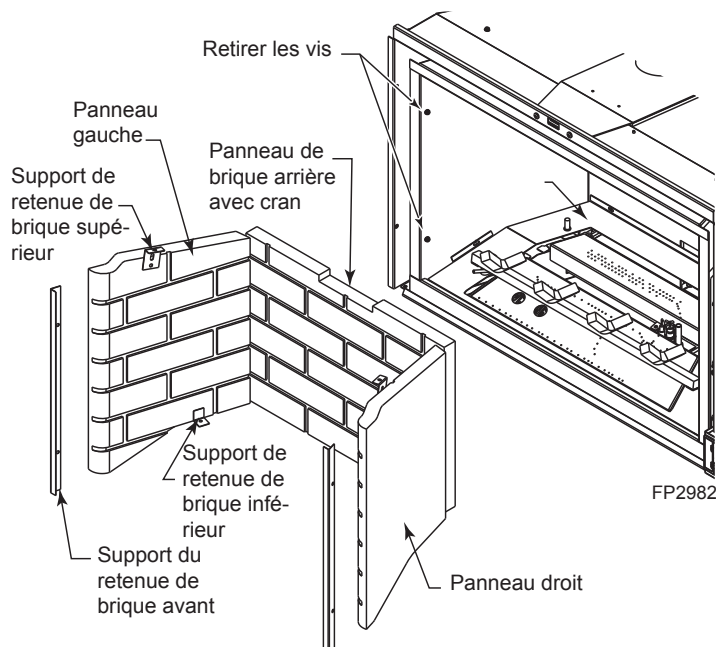
Figure 13 - Installer de panneaux des briques
