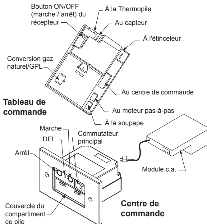
Figure 35 - Composants du système de commande Signature
