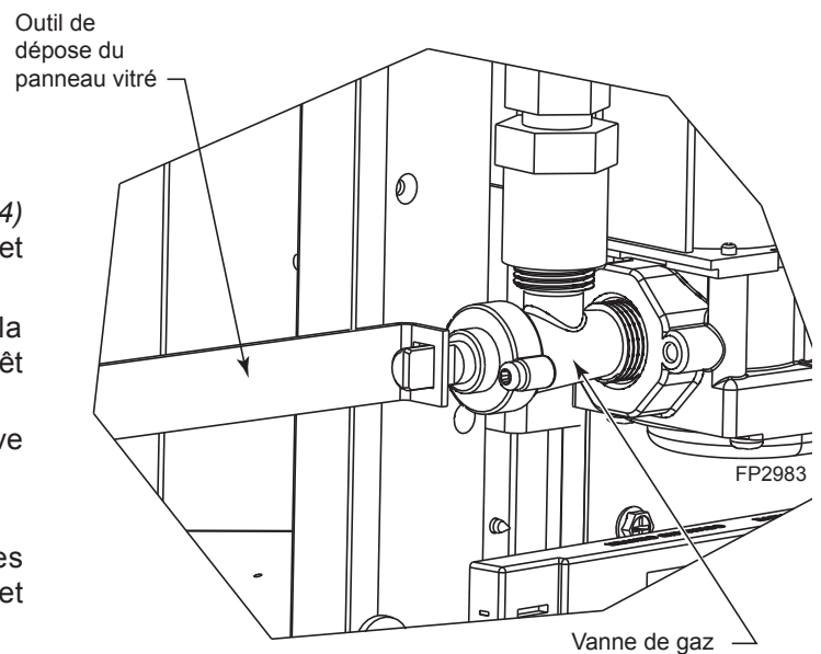
Figure 21 - Utilisez l'outil de dépose du panneau vitré pour couper l'alimentation en gaz
