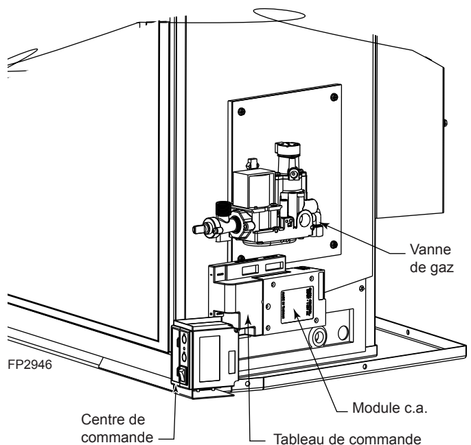
Figure 1 - Contrôles du foyer encastrable VC41LDVI.
