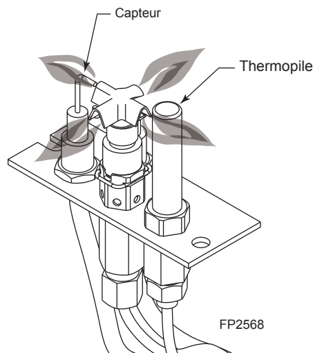
Figure 52 - Avant de démonter l'appareil, vérifiez la flamme de la veilleuse. La flamme devrait toucher au thermocouple et à la thermopile
