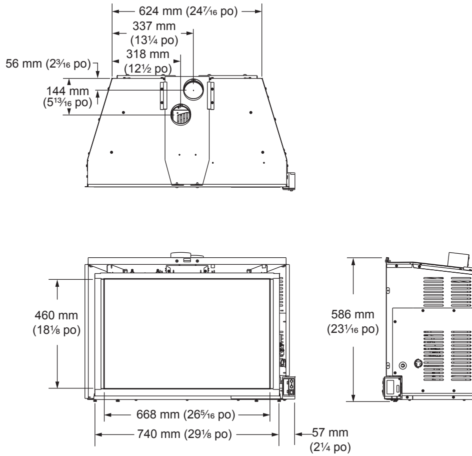
Figure 2 - Dimensions du foyer encastrable
