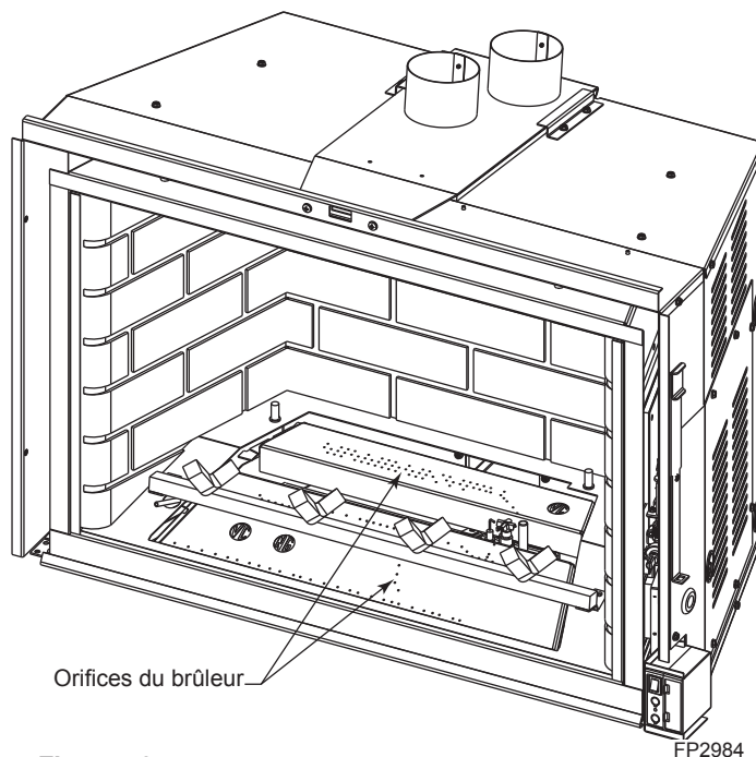
Figure 53 - Vérification des orifices du brûleur et des brûleurs
