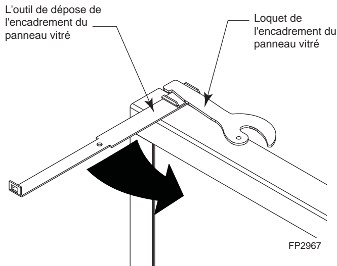
Figure 15 - Utilisez un outil (fourni) pour dégager les loquets de l'encadrement
