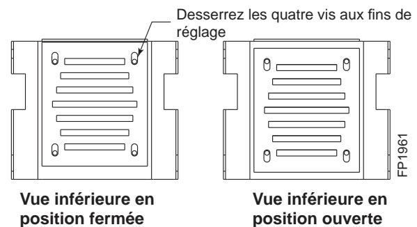
Figure 14 - Ensemble de chicane et réglage
