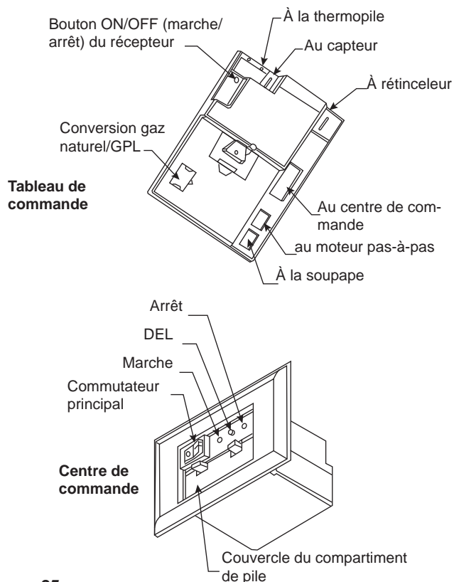
Figure 35 - Composants du système de commande Signature
