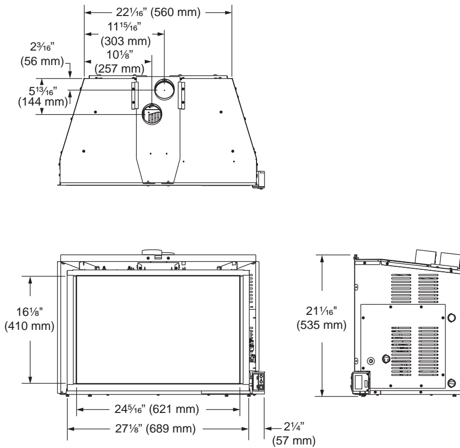
Figure 2 - Dimensions du foyer encastrable
