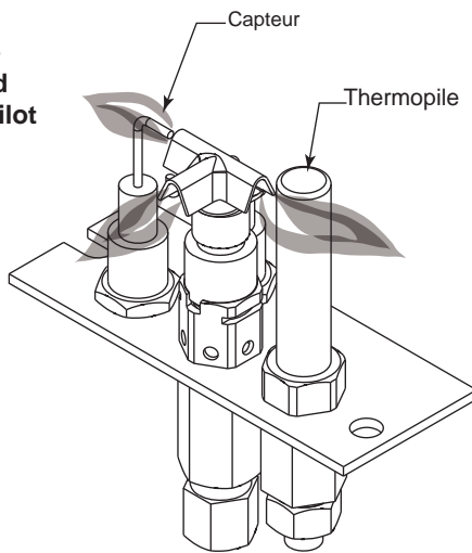
Figure 53 - Avant de démonter l'appareil, vérifiez la flamme de la veilleuse. La flamme devrait toucher au thermocouple et à la thermopile
