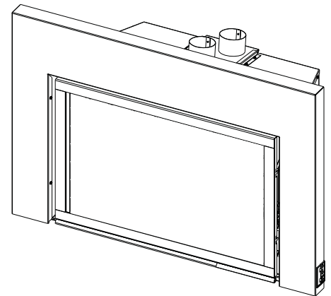
Figure 33 - Petit encadrement avec accès de commande centre latéral
