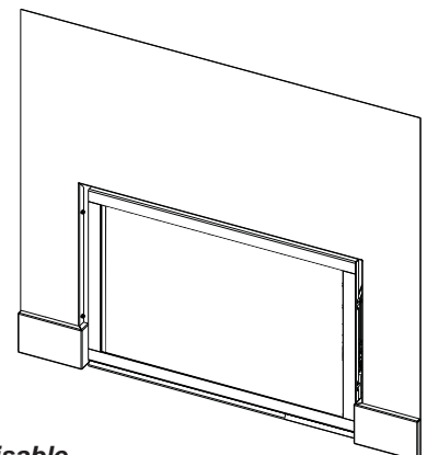
Figure 33 - Petit encadrement avec accès de commande centre latéral
