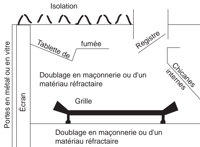
Figure 8 - Exigences pour les foyers en métal à dégagement nul
