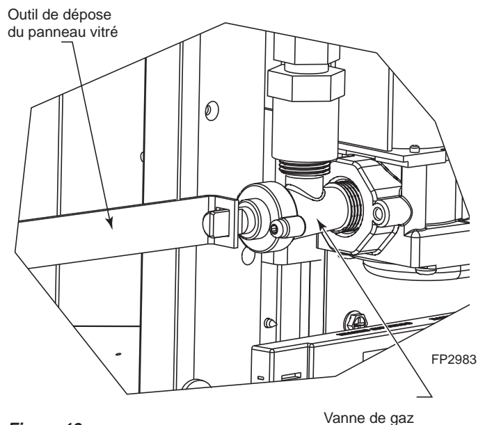
Figure 19 - Utilisez l'outil de dépose du panneau vitré pour couper l'alimentation en gaz
