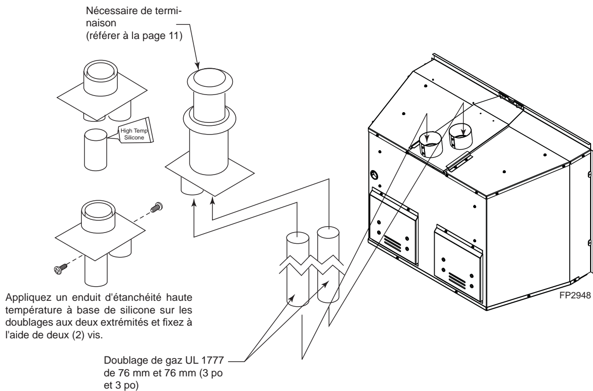
Figure 10 - Raccordement du tuyau de ventilation à l'appareil de chauffage
