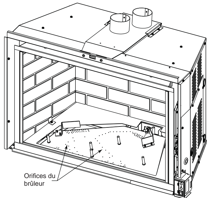
Figure 54 - Vérification des orifices du brûleur et des brûleurs
