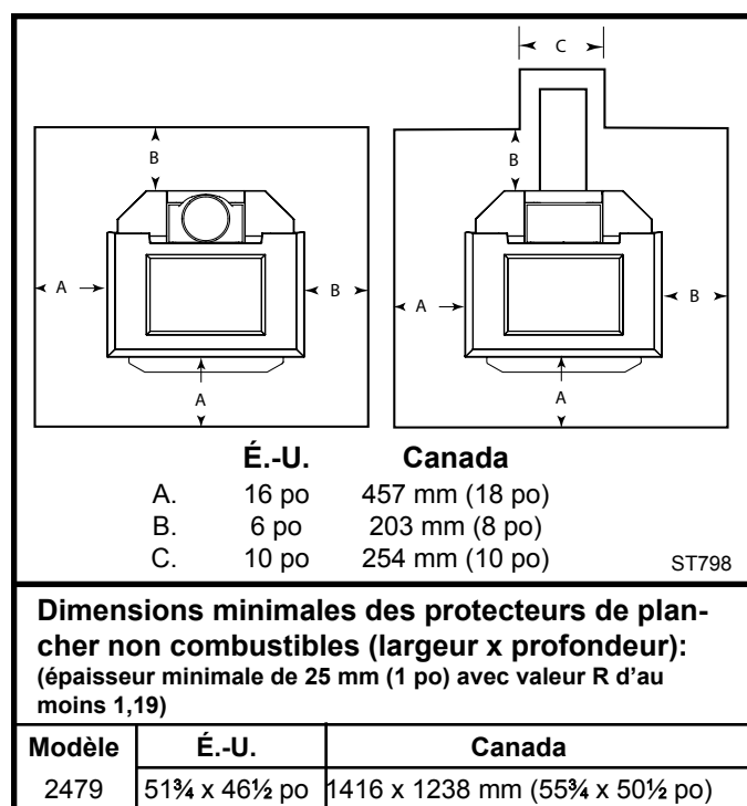
Fig. 12 Assurez-vous de répondre aux exigences minimales relatives à la protection du plancher sur les quatre côtés du poêle.
