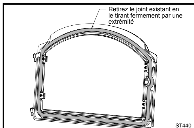
Fig. 32 Joint de porte.
