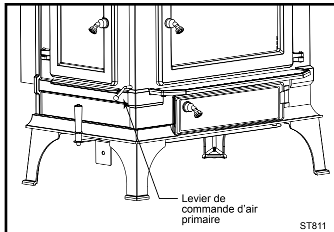
Fig. 25 Pour ouvrir, tournez le levier de commande dans le sens horaire.
