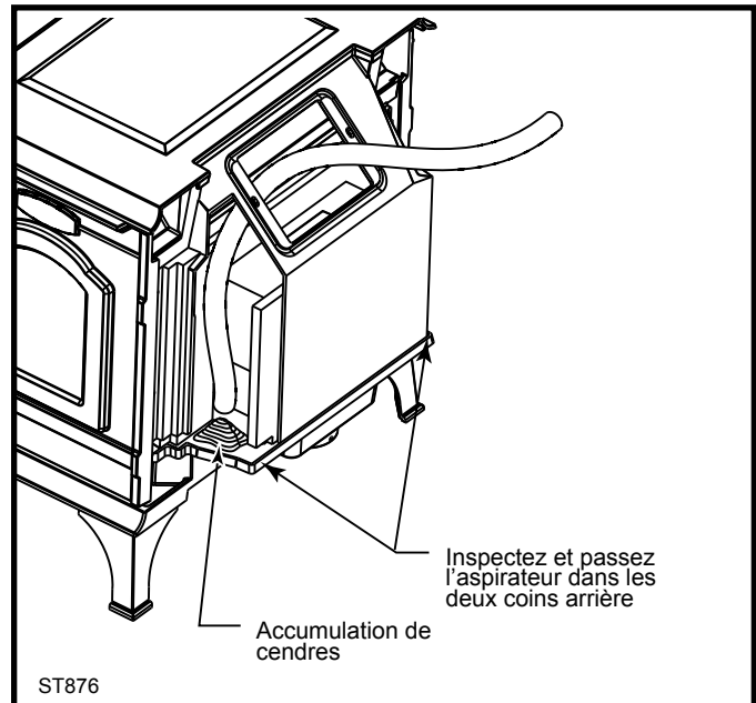
Fig. 35 Inspectez et nettoyez l'accumulation de cendres sur chaque côté du système de combustion non-catalytique.
