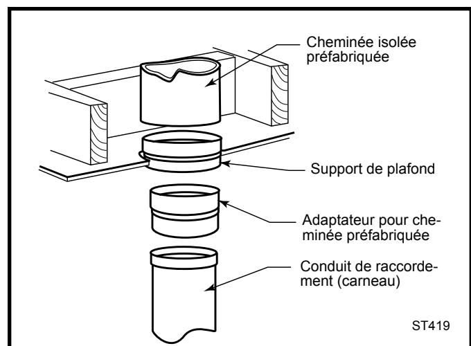
Fig. 6 Raccordement d'un carneau à une cheminée préfabriquée.
