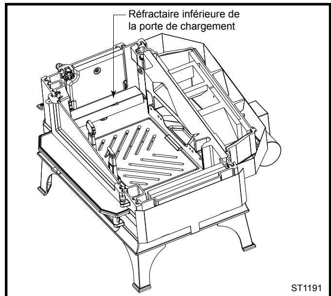
Fig. 22 Installer le réfractaire inférieure de la porte. (Vue en coupe d'éclaircissement.)
