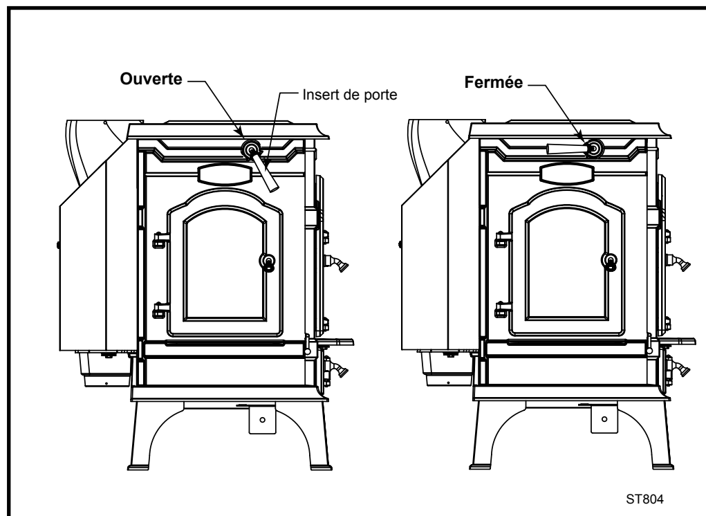
Fig. 27 Positions du registre.
