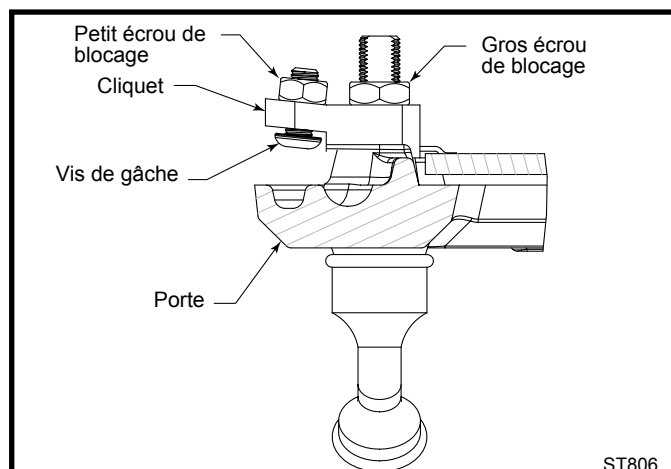
Fig. 31 Ajustement du verrou de porte.
