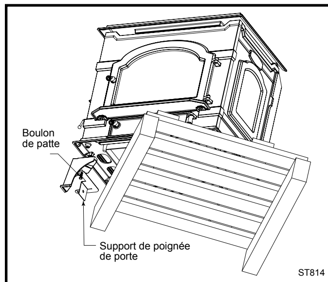
Fig. 20 Tournez le poêle sur la palette pour exposer le coin avant gauche.
