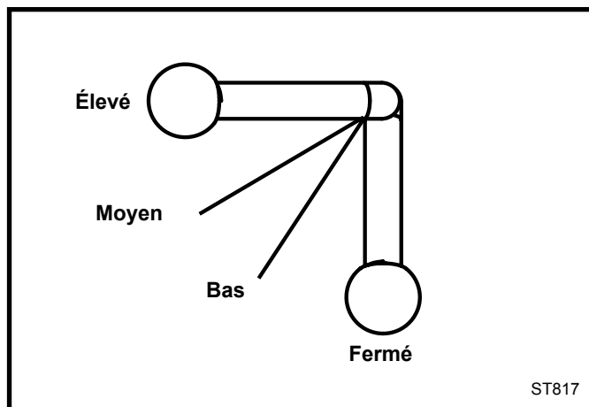
Fig. 28 Réglez le levier de commande d'air primaire pour obtenir des taux de combustion différents.
