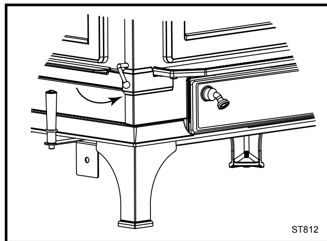
Fig. 26 Pour fermer, tournez le levier de commande dans le sens antihoraire.
