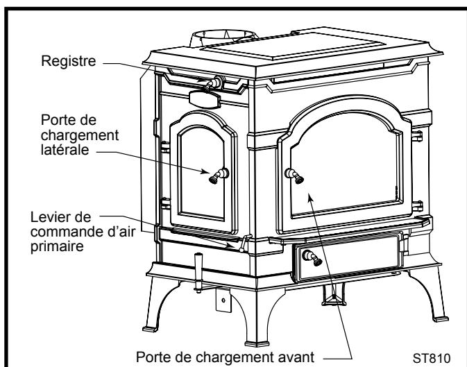
Fig. 24 Commandes du poêle.
