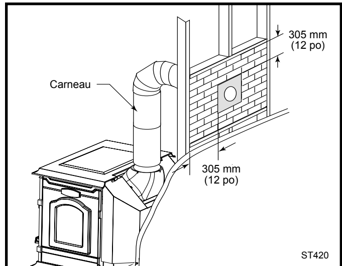
Fig. 10 Passe-mur avec matériaux non combustibles.
