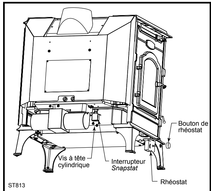
Fig. 23 Fan installation.
