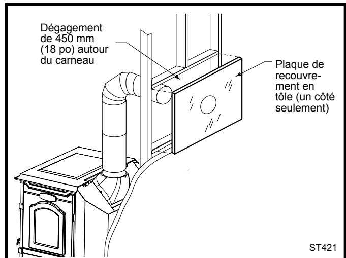
Fig. 11 Passe-mur creux.
